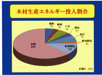
②木材生産のためのエネルギー投入割合
