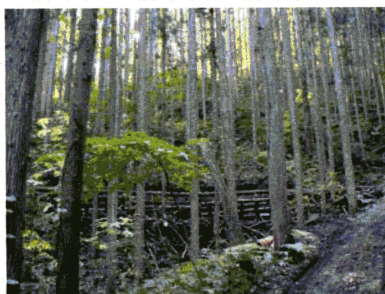
⑩超高密度作業路網
