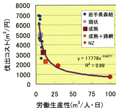
⑪労働生産性とコスト(1)
